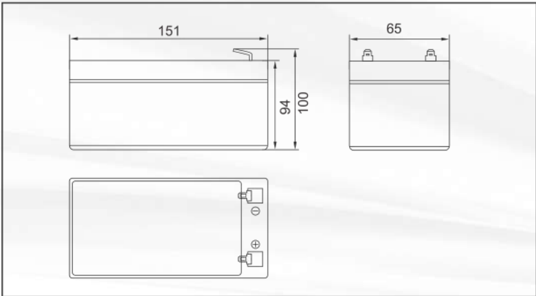
DIMENSÕES EXTERNAS
